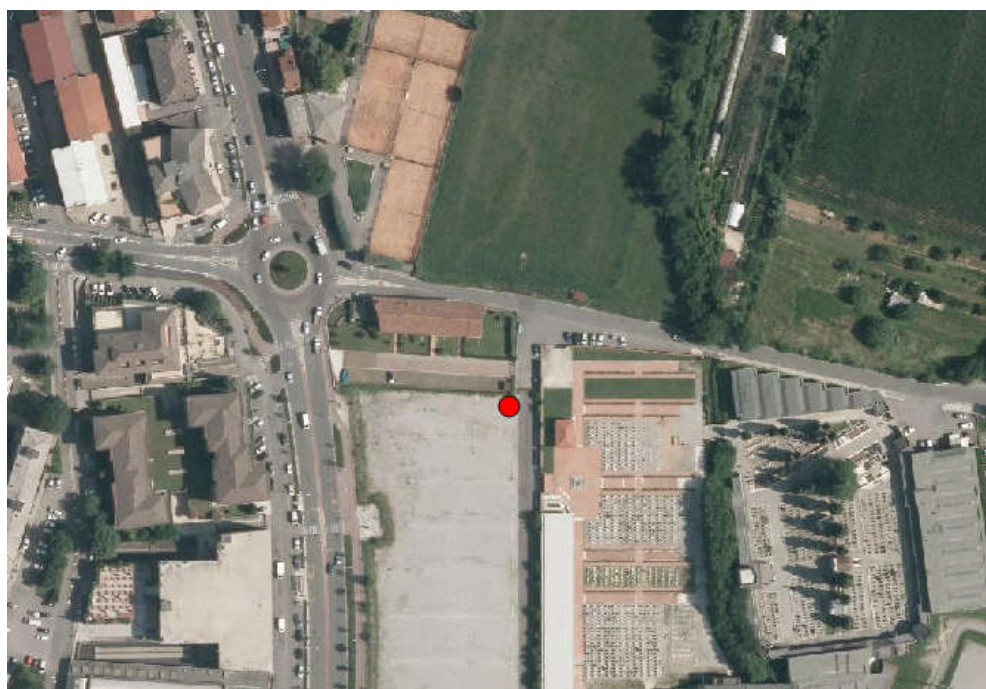
Figura 6 - Ubicazione piezometro BS002_MW14 Coordinate Gauss-Boaga X: 1596194 Y: 5047306
