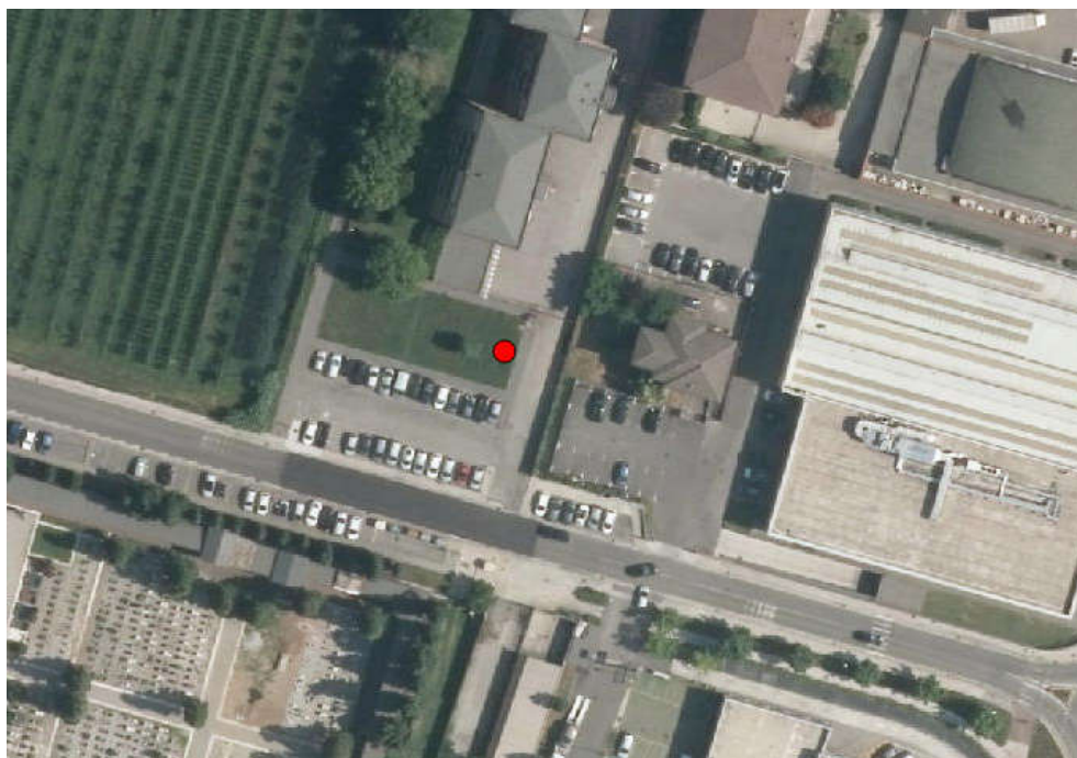
Figura 7 - Ubicazione piezometro BS002_MW15 Coordinate Gauss-Boaga X: 1595941 Y: 5046886
