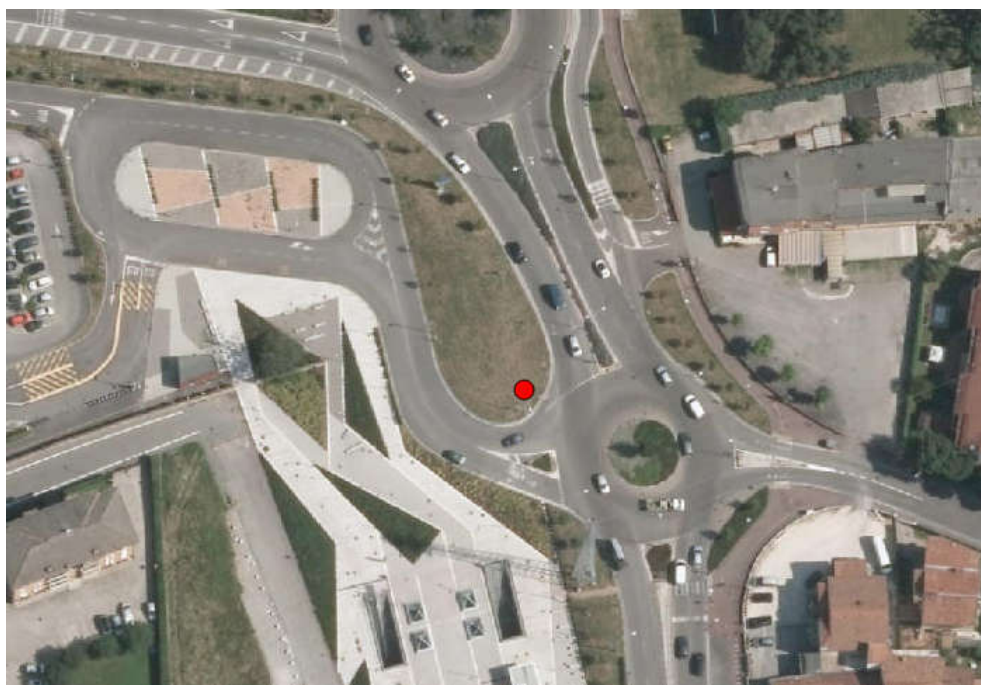
Figura 5 - Ubicazione piezometro BS002_MW13 Coordinate Gauss-Boaga X: 1595932 Y: 5048170
